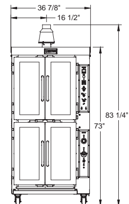
JAOP6G Front
