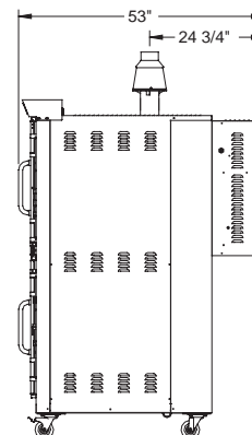
JAOP6G Side
